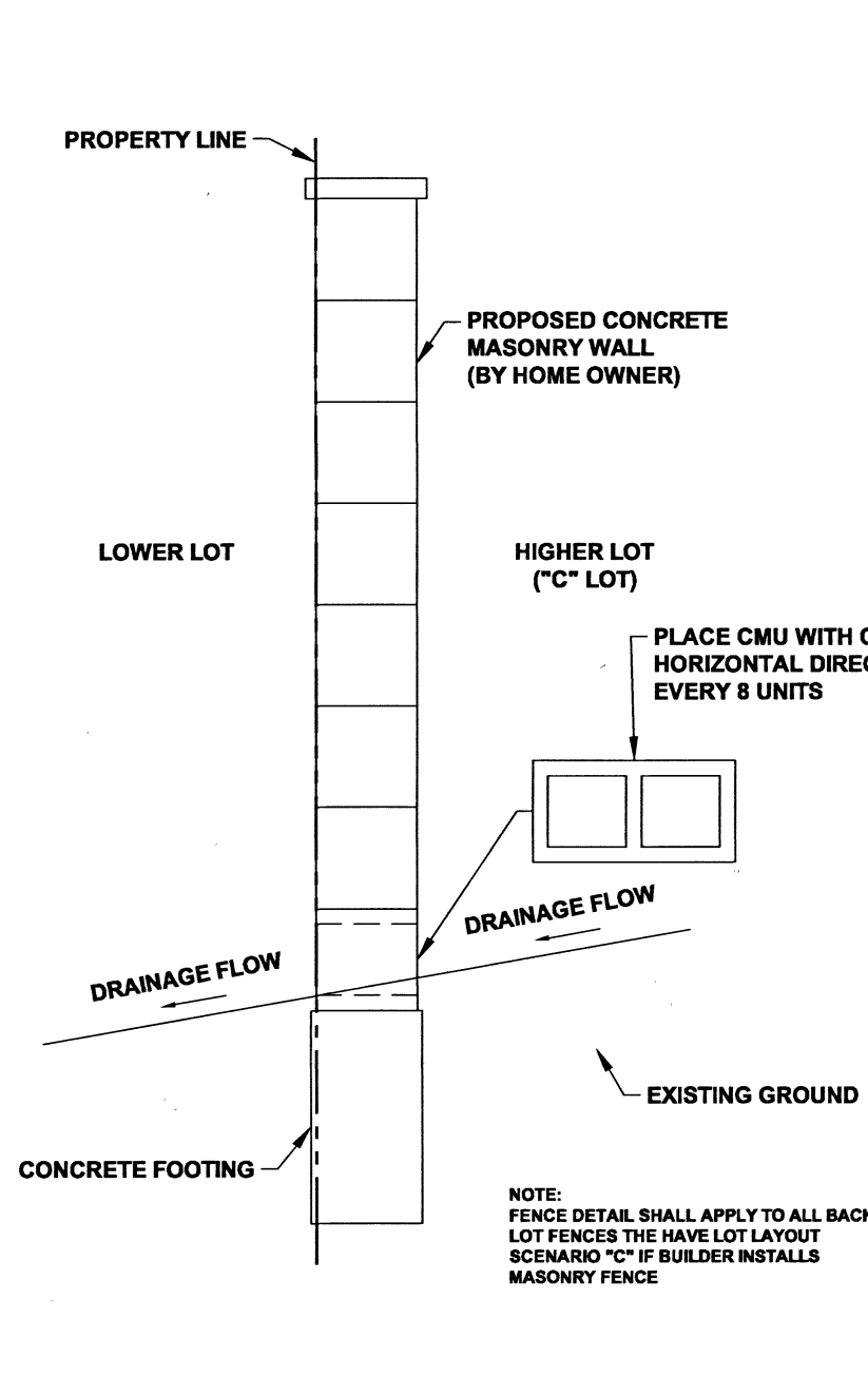
4 CONCRETE MASONRY WALL DETAIL SCALE: N.T.S.
