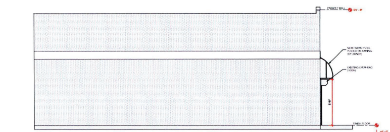
4 ELEVATION SCALE: 3/16" = 1'-0"
